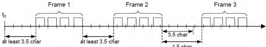
Abbildung 2: 3,5 Zeichen Timeout zwischen Frames (MB Ser Spec Kap. 2.5.1.1)
